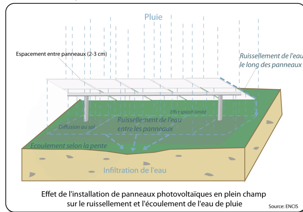
Figure 14 : Effet d'une installation photovoltaïque en plein champ sur l'écoulement de l'eau de pluie (source : ENCIS Environnement)
