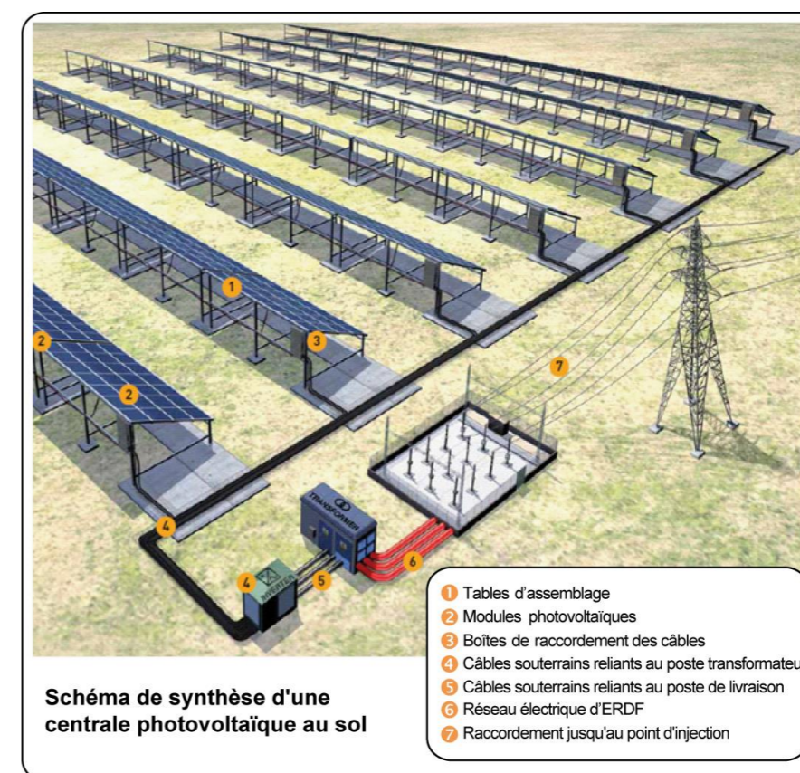
Figure 19 : Schéma d'une centrale photovoltaïque.
