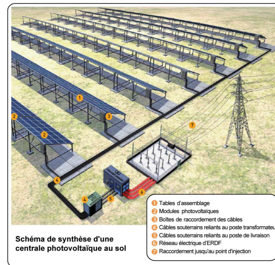
Figure 9 : Schéma d'une centrale photovoltaïque.
