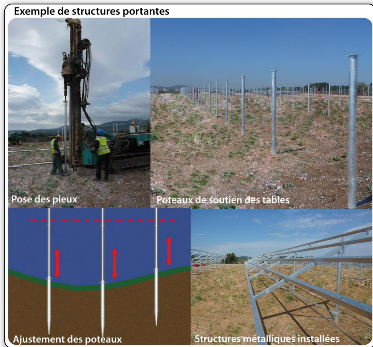
Figure 16 : Structures porteuses métalliques (Source : ENCIS Environnement)
